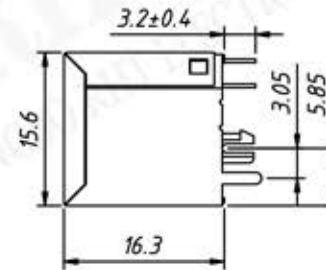
A-A 4:1
