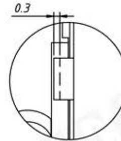
A-A 4:1
